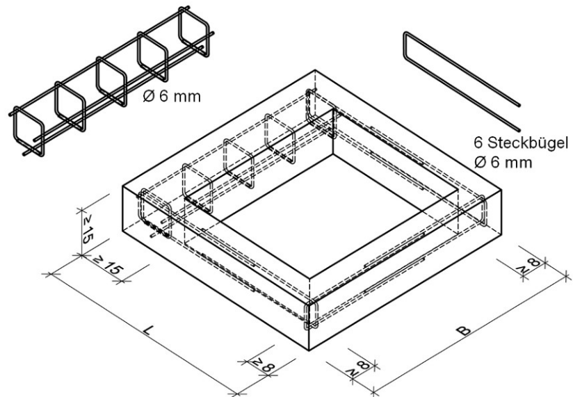
Bild 16 Mindestabmessungen
