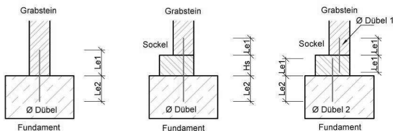
Bild 3 Verdübelung
