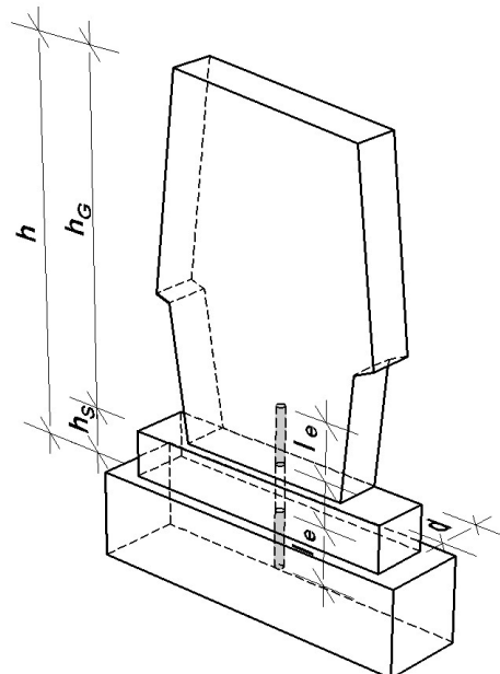
Bild 2 Verdübelung
